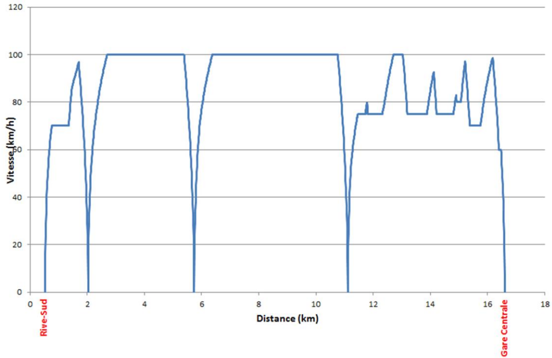
Profil de vitesse - Direction Gare Centrale
